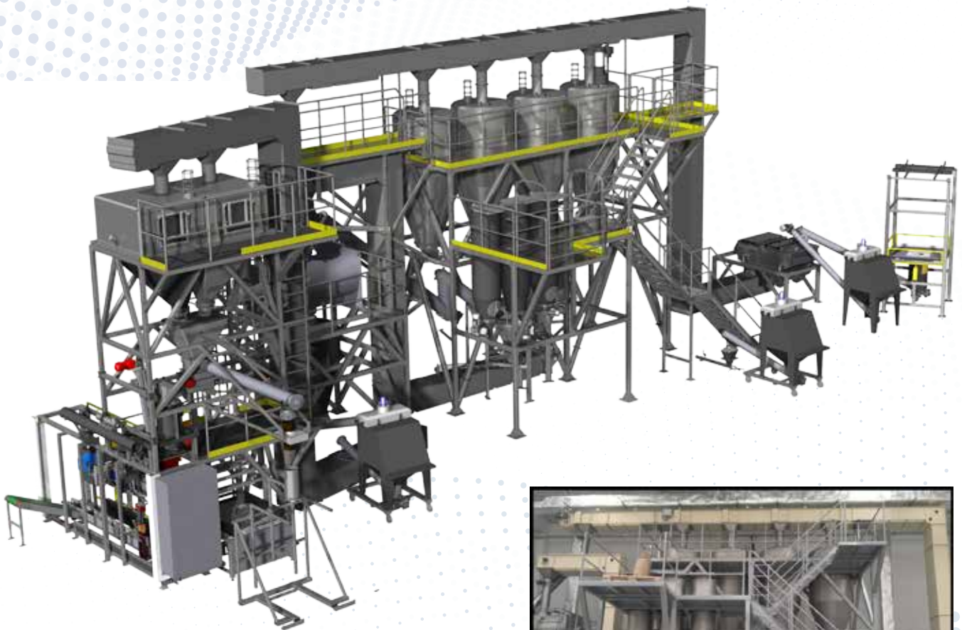
Visualisation d'une usine existante de production de mélanges laitiers.
