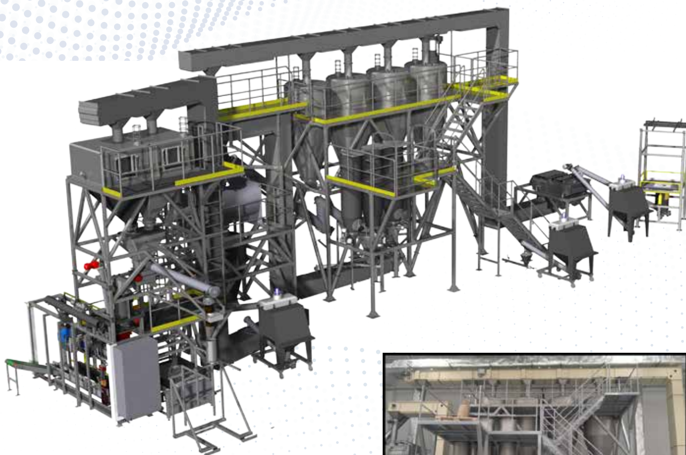
Przykładowa wizualizacja istniejącej wytwórni mieszanek mlecznych.
