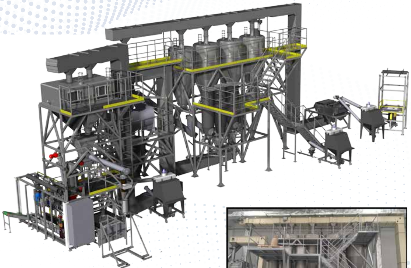
Beispielhafte Visualisierung einer bestehenden Milchmischanlage.
