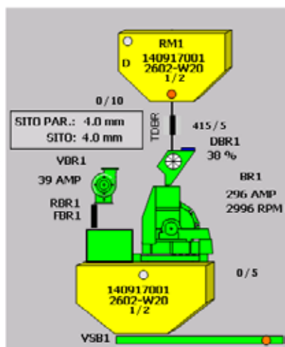
Linia mielenia z regulacją obciążenia młynka oraz kontrolą sit control
